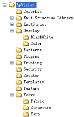
图 1-13 目录结构图
